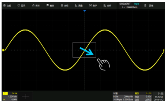
通过单点拖动手指绘制矩形框，手指移开屏幕出现菜单，可选择区域触发、直方图功能。在手势开始时请保持角度在 45^\circ 左右以保证仪器能正确识别为画框操作
